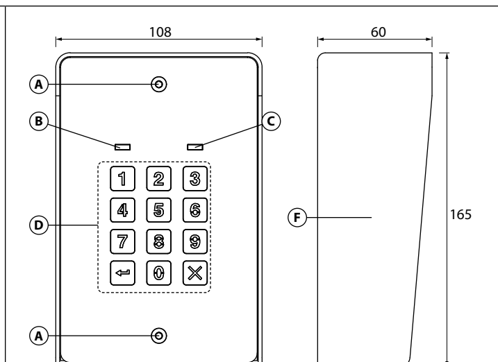
Fig. 2 Art. VX8901S - Montaggio da superficie
