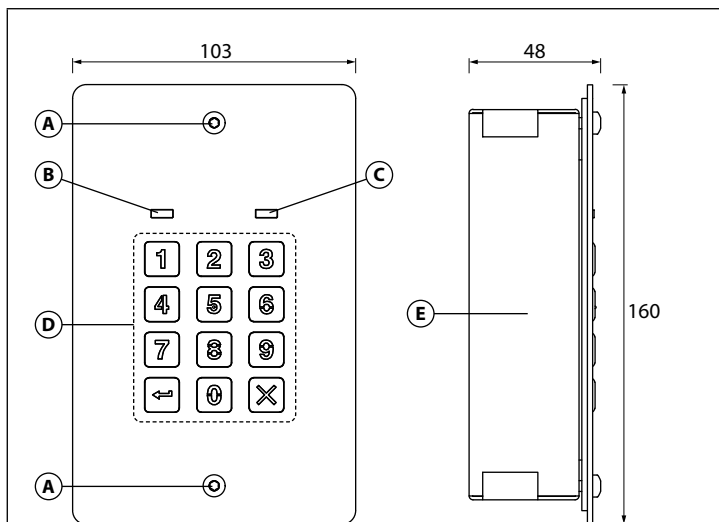
Fig. 1 Art. VX8901F - Montaggio da incasso
